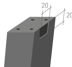
Detail s kótami otvorů
