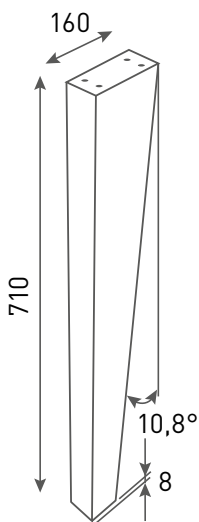
Schéma nohy s kótami
